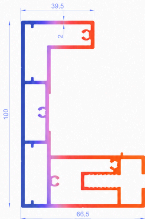
T.2479 - 2,718 кг/м ФИКСИРАН ВЕРТИКАЛЕН ПРОФИЛ
