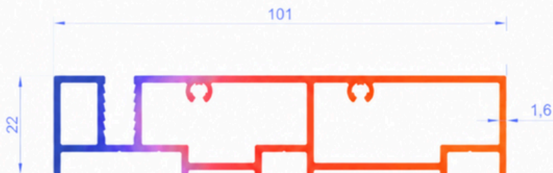
T.2481 - 1,472 кг/м ФИКСИРАН ХОРИЗОНТАЛЕН ПРОФИЛ
