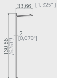
Капак за стенен профил
