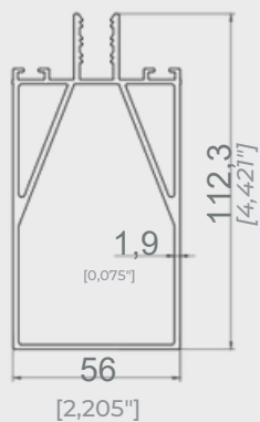
Носещ профил за стъкло
