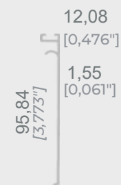
Капак за стена и улук
