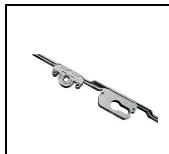
OPT-2018 Slide Espagnolette 160cm with Barrel
