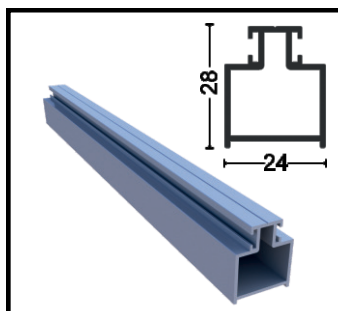
OPT-1014-50 Sidebar Profile
