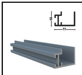
SRM-1010 Puller Profile (10 mm) Weight 0.144 kg/m
