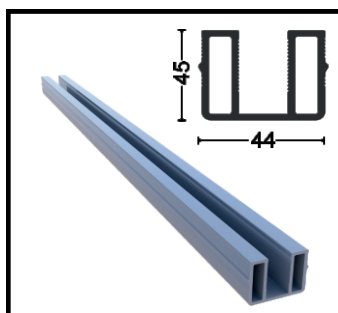
OPT-1017-60 8mm Adapter Profile
